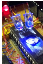
EPROM(UVEPROM)
